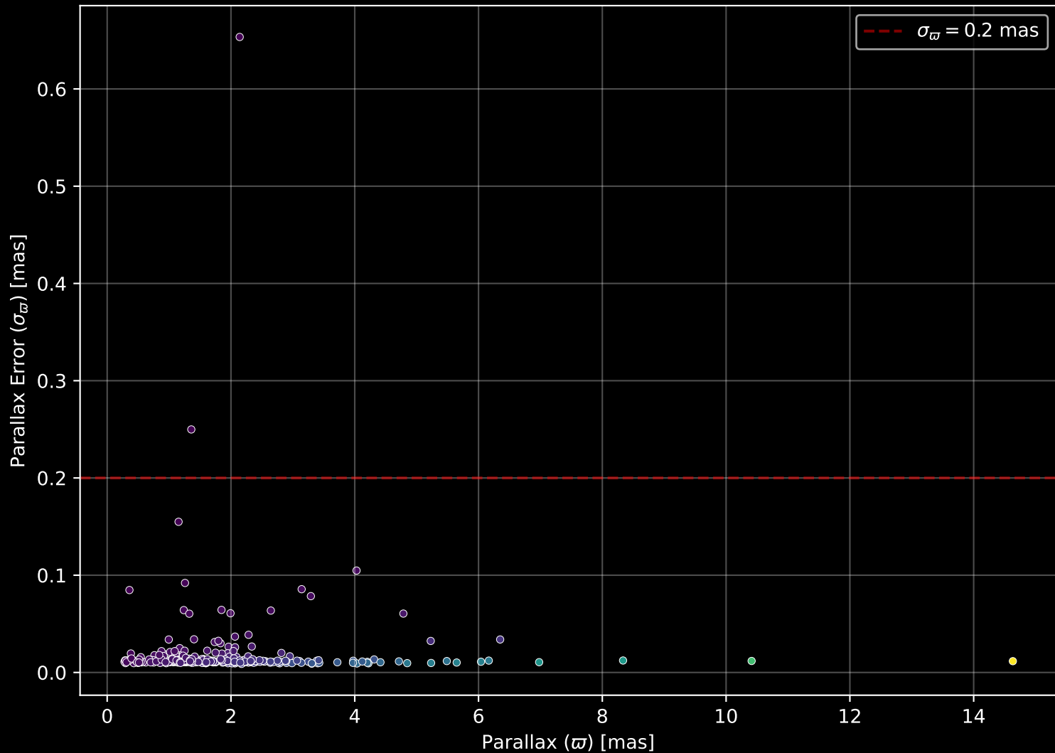
GALAH DR4 Field: [556] Parallax Quality (n= 310)
