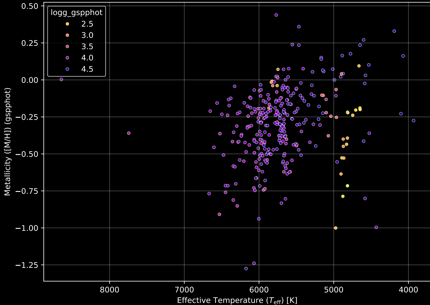
GALAH DR4 Field: [556] Stellar Population Parameters (n= 310)
