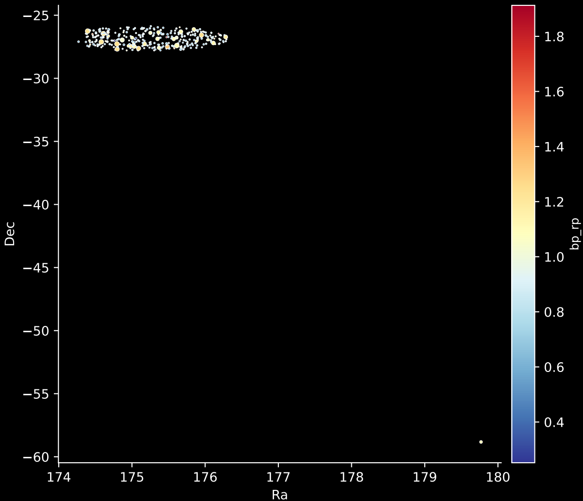
GALAH DR4 Field: [556] Stars: 310
