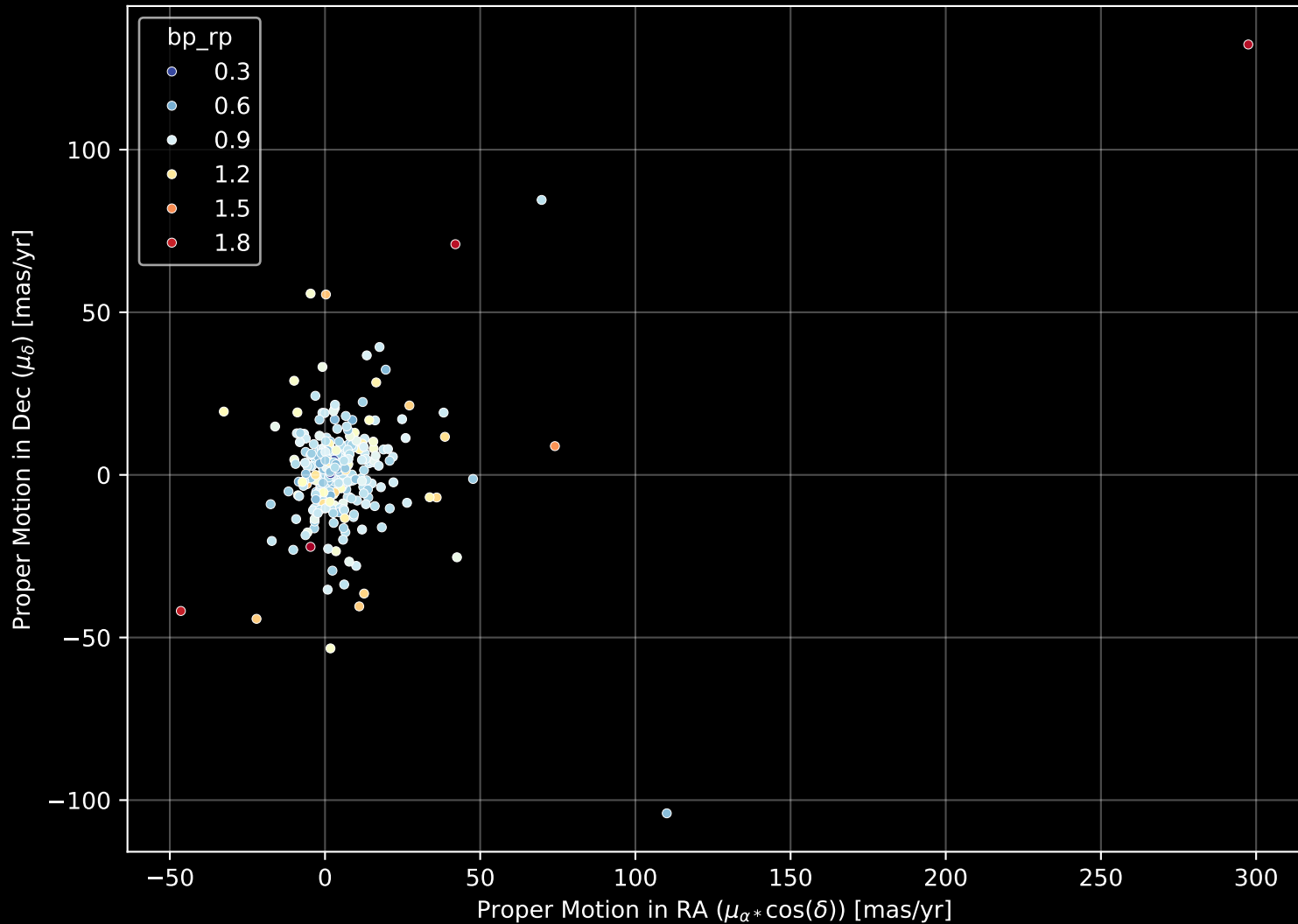
GALAH DR4 Field: [556] Proper Motion Diagram (n= 310)
