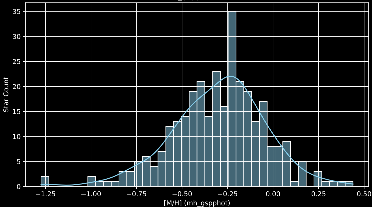
GALAH DR4 Field: [556] [M/H] (mh_gspphot) (n= 310)
